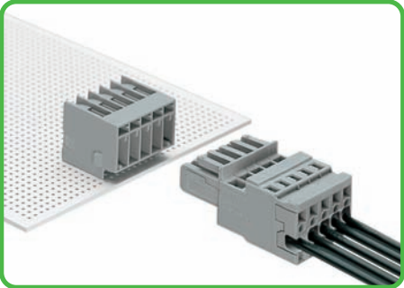
Монтажный блок с выводами под пайку углового исполнения
