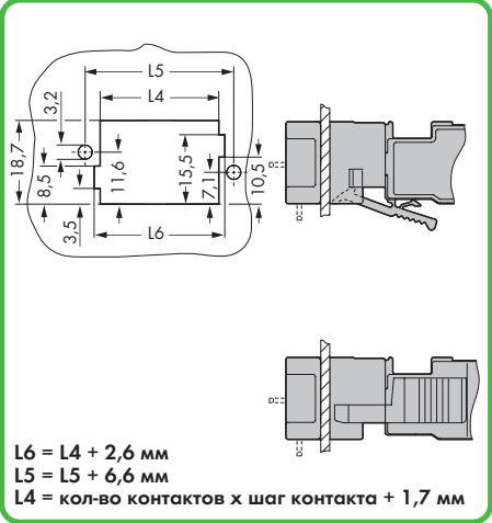
Отверстие для монтажного блока
